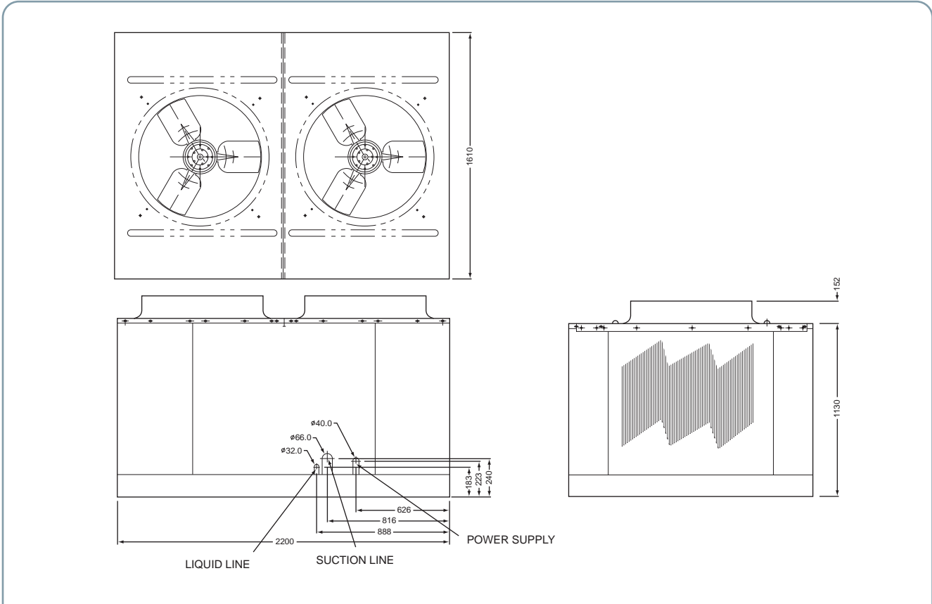
Model : 38AE020-040
